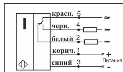
Схема соединения
