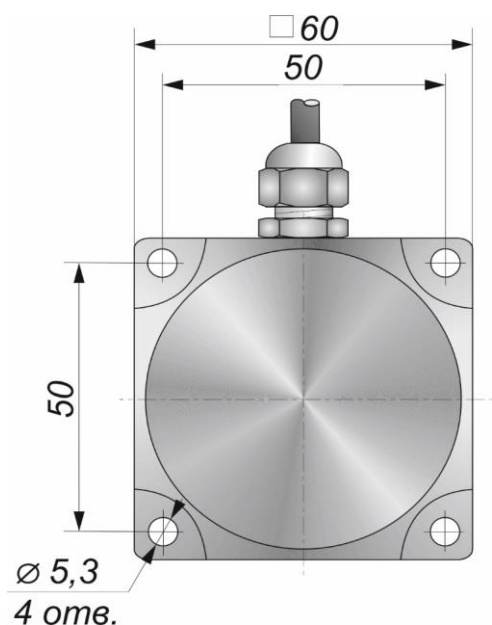
Габаритный чертеж
