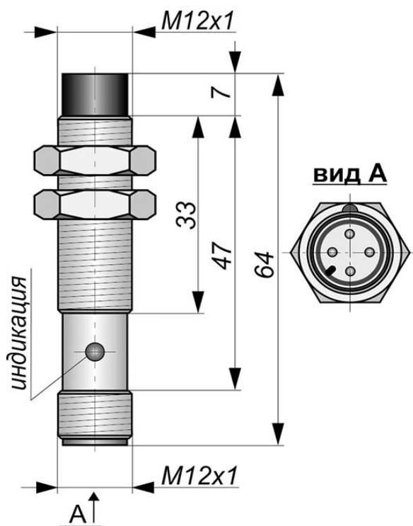
Габаритный чертеж
