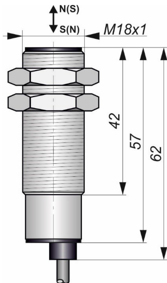
Габаритный чертеж
