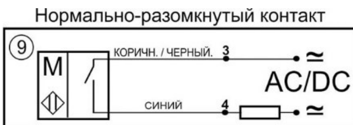
Схема соединения
