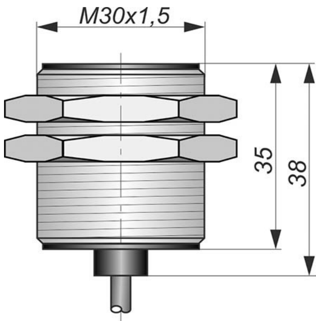
Габаритный чертеж
