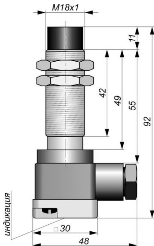
Габаритный чертеж
