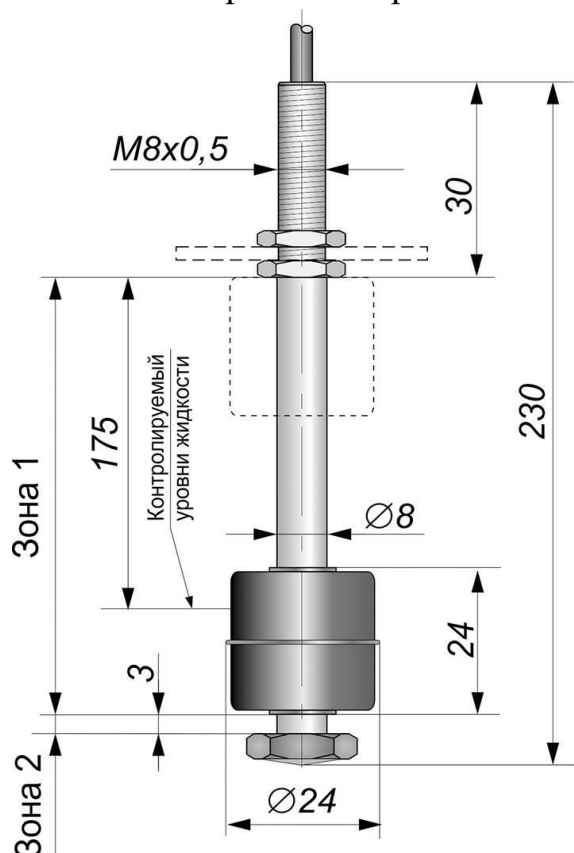
Габаритный чертеж
