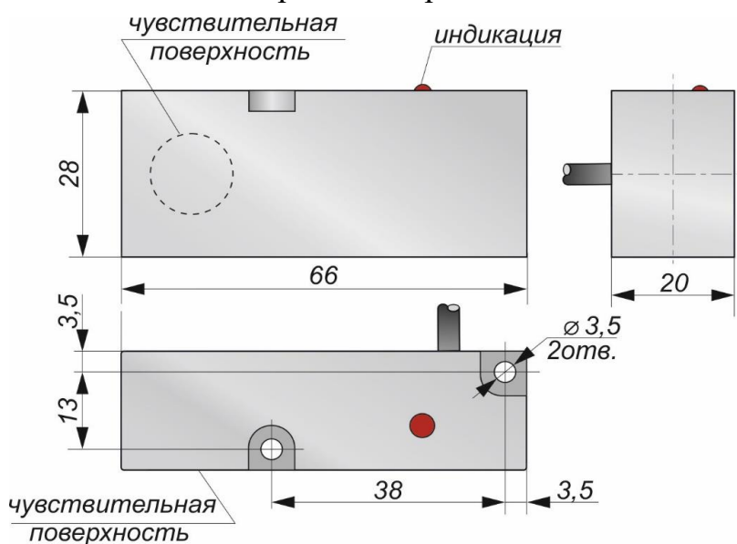
Габаритный чертеж
