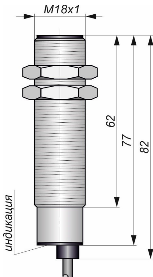
Габаритный чертеж
