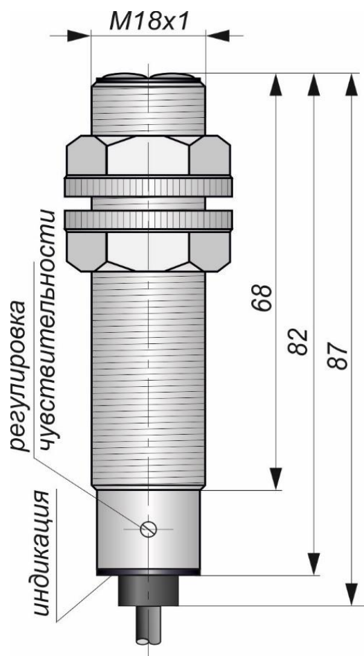
Габаритный чертеж
