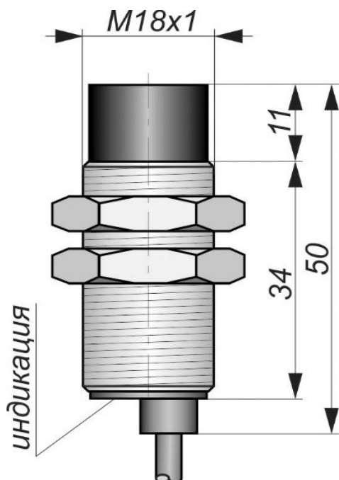
Габаритный чертеж
