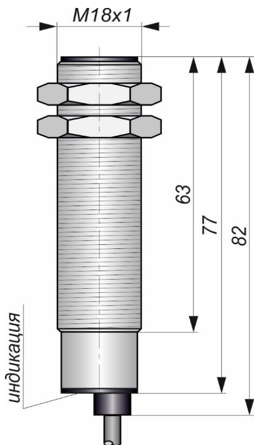
Габаритный чертеж
