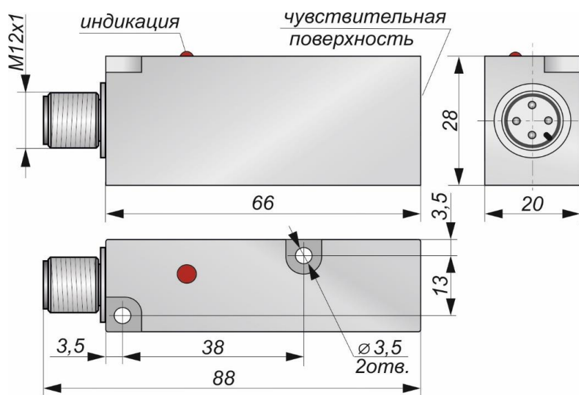
Габаритный чертеж
