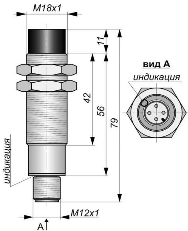
Габаритный чертеж
