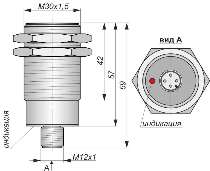
Габаритный чертеж
