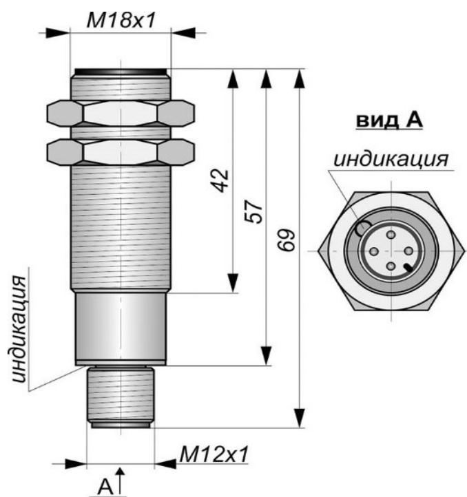
Габаритный чертеж
