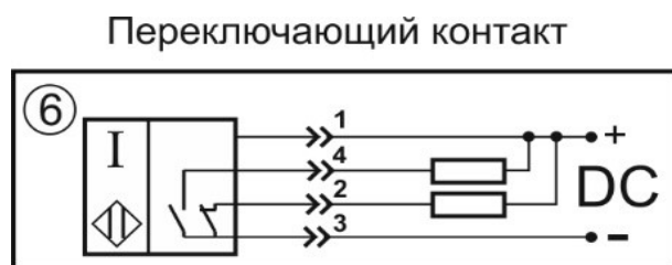
Схема соединения
