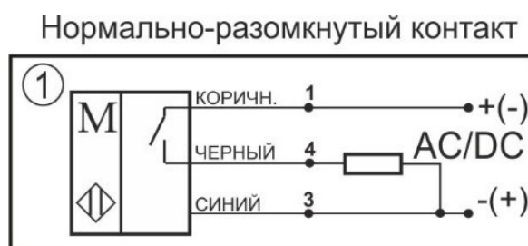
Схема соединения
