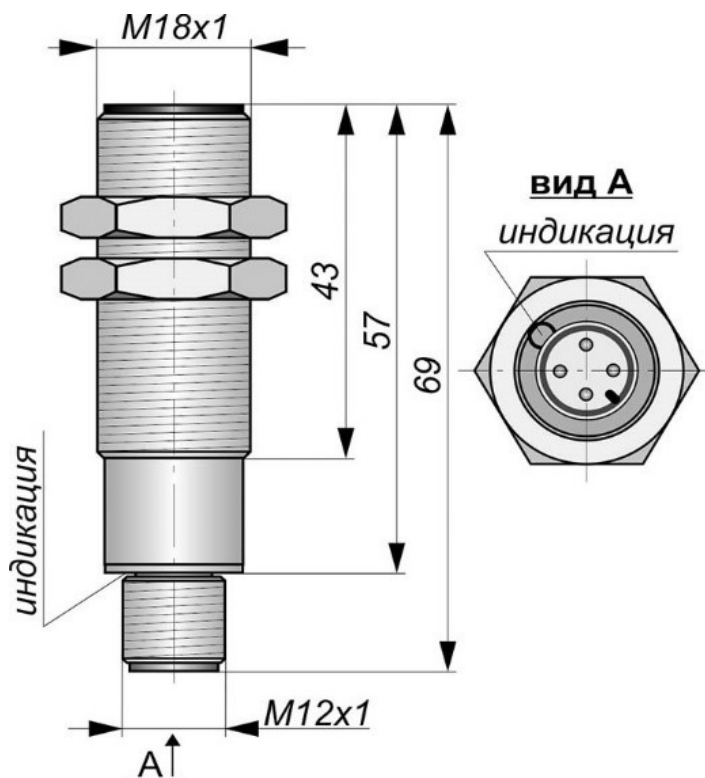
Габаритный чертеж
