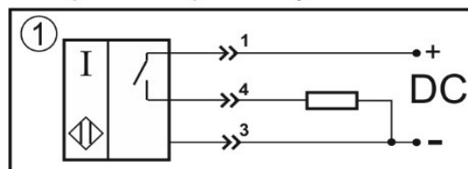
Цоколевка разъема
