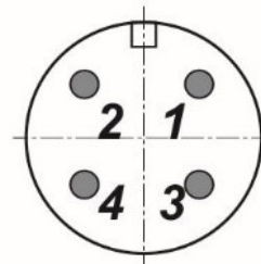
Цоколевка разъема
