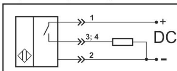
Цоколевка разъема
