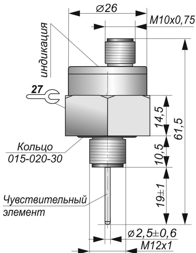
Габаритный чертеж
