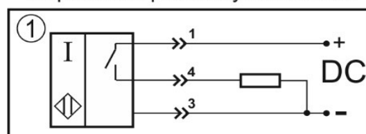
Цоколевка разъема
