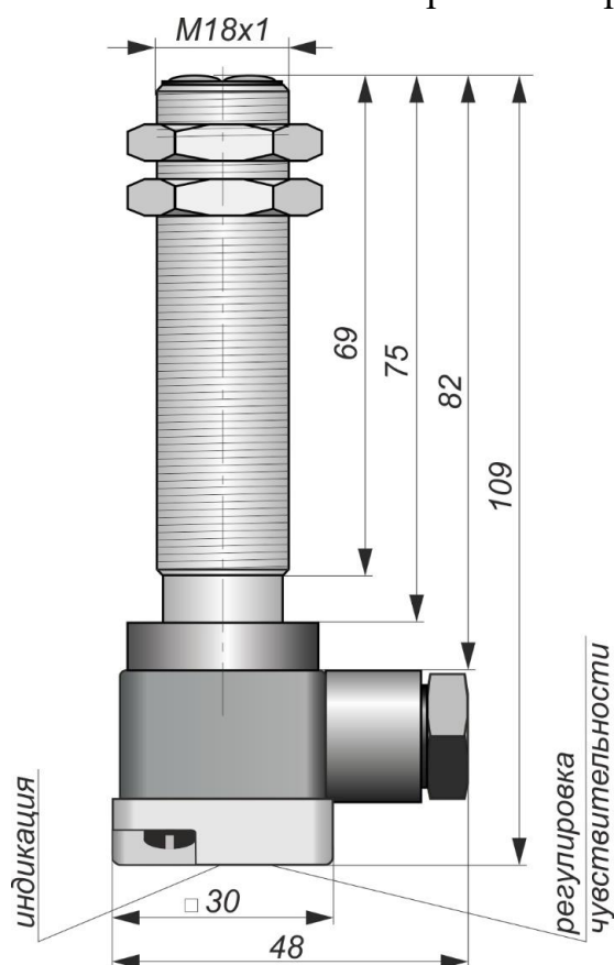
Габаритный чертеж
