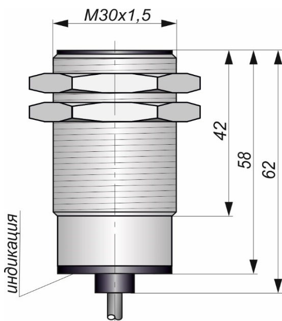
Габаритный чертеж
