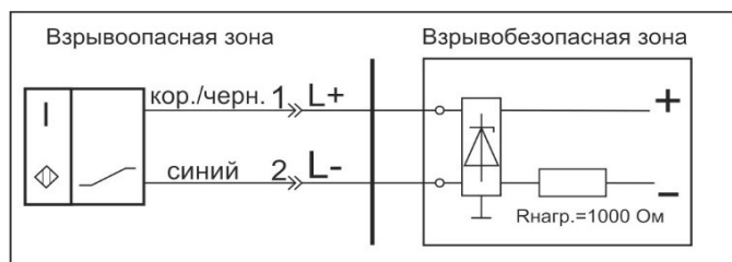
Схема соединения
