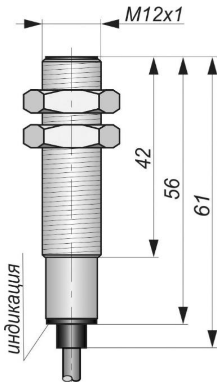
Габаритный чертеж
