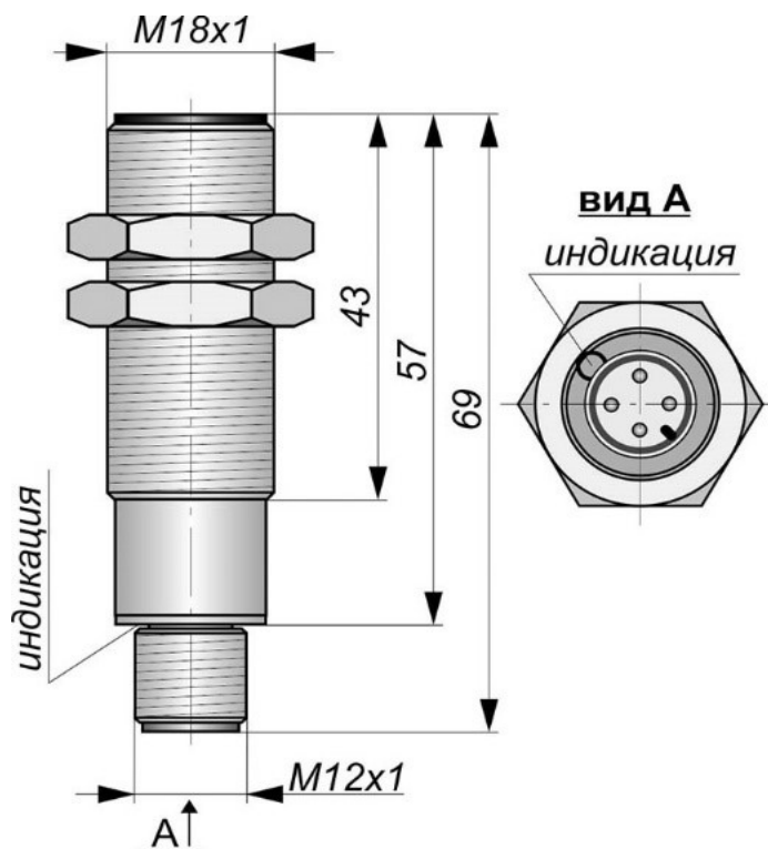
Габаритный чертеж
