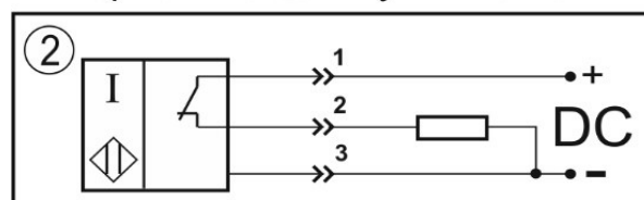
Цоколевка разъема
