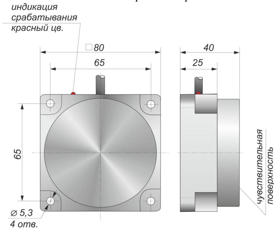
Габаритный чертеж
