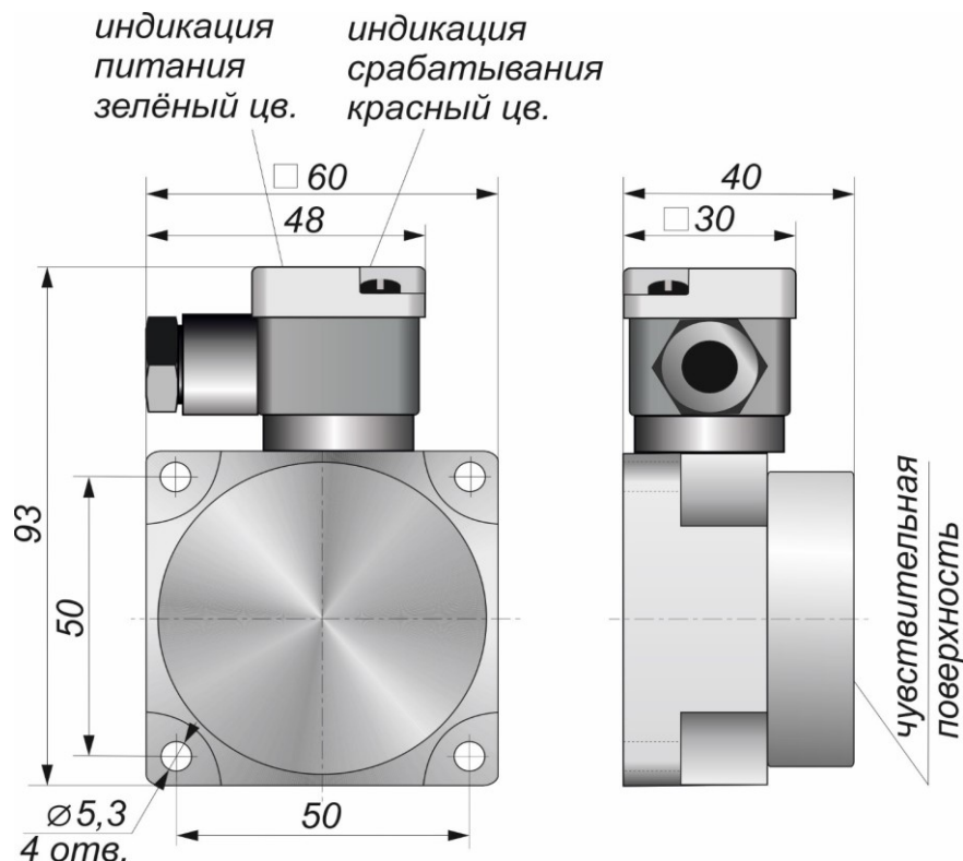
Габаритный чертеж
