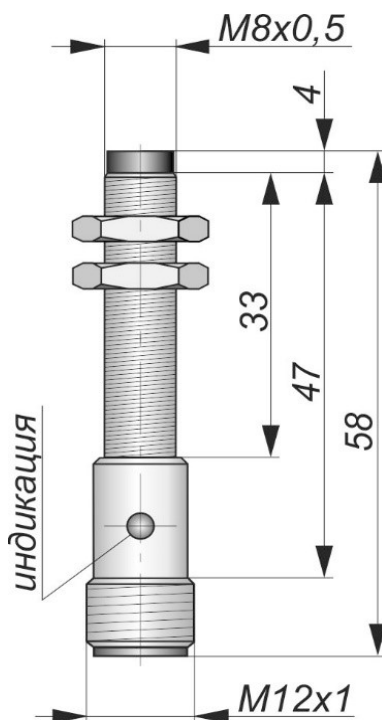
Габаритный чертеж
