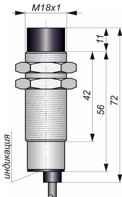
Габаритный чертеж
