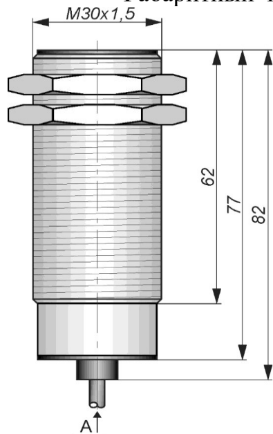
Габаритный чертеж
