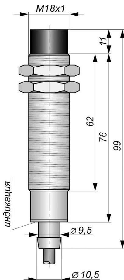
Габаритный чертеж
