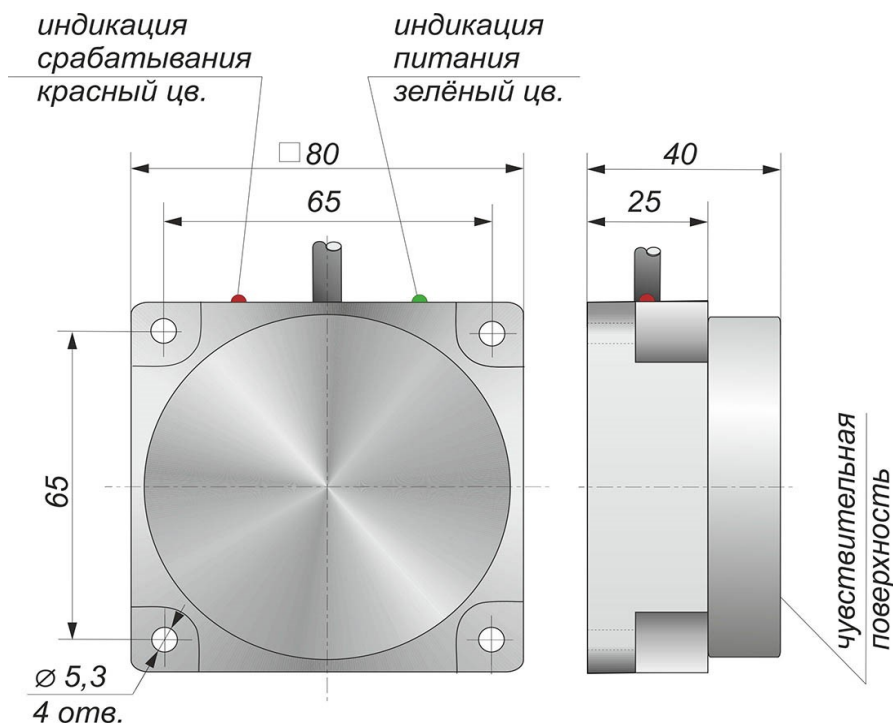
Габаритный чертеж
