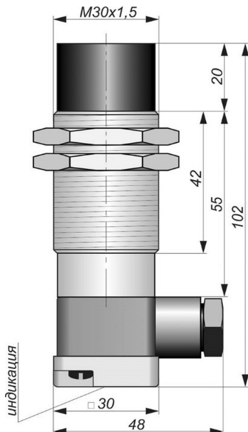
Габаритный чертеж
