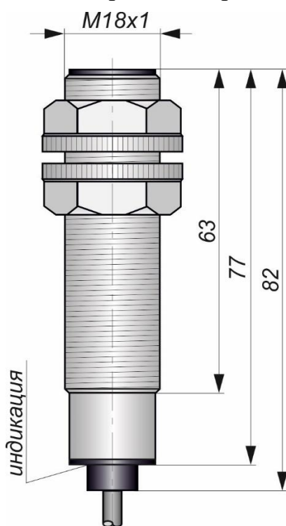
Габаритный чертеж
