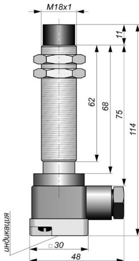
Габаритный чертеж
