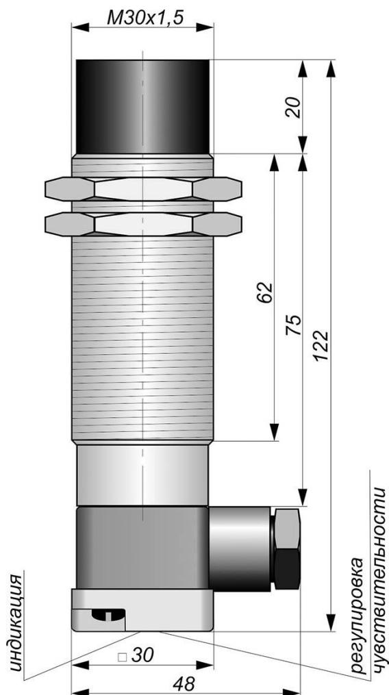
Габаритный чертеж
