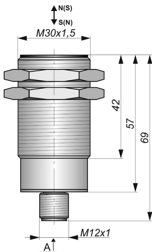
Габаритный чертеж
