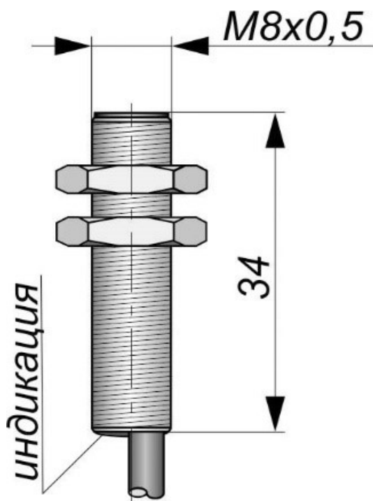
Габаритный чертеж
