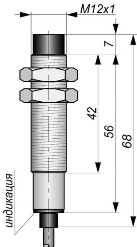
Габаритный чертеж
