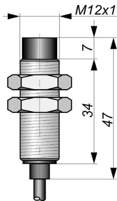
Габаритный чертеж
