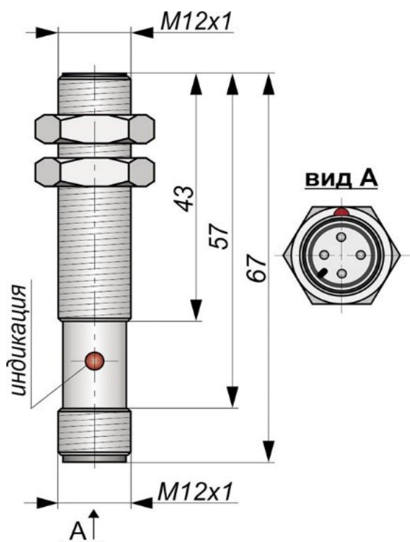
Габаритный чертеж
