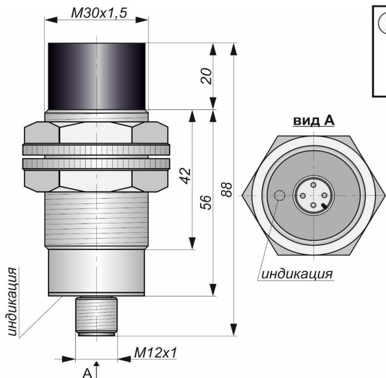
Габаритный чертеж
