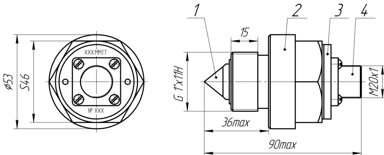
Рисунок 1 — Конструкция датчика
