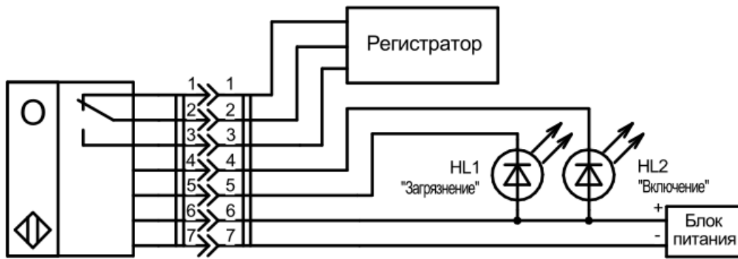
Рисунок 2 — Схема подключения датчика
