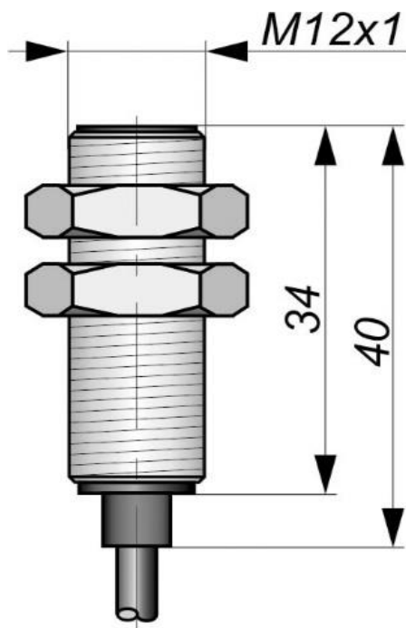
Габаритный чертеж
