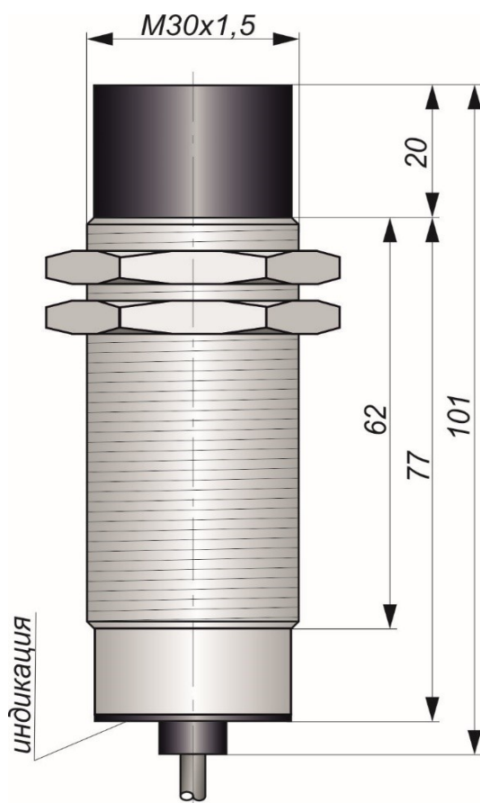
Габаритный чертеж
