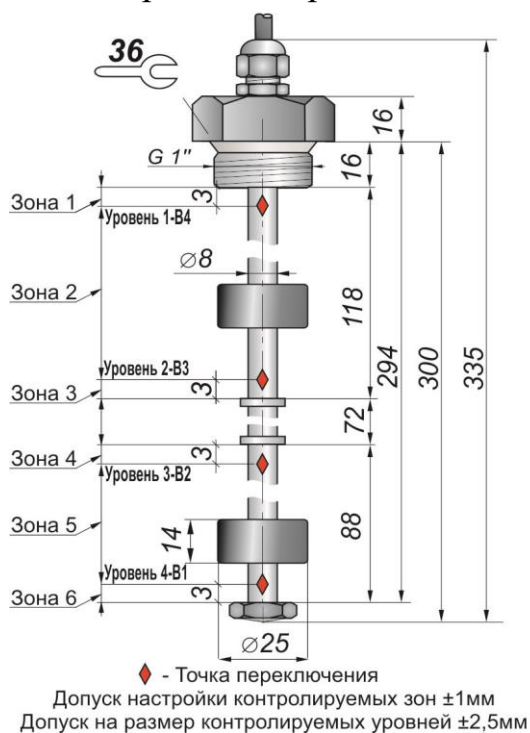
Габаритный чертеж
