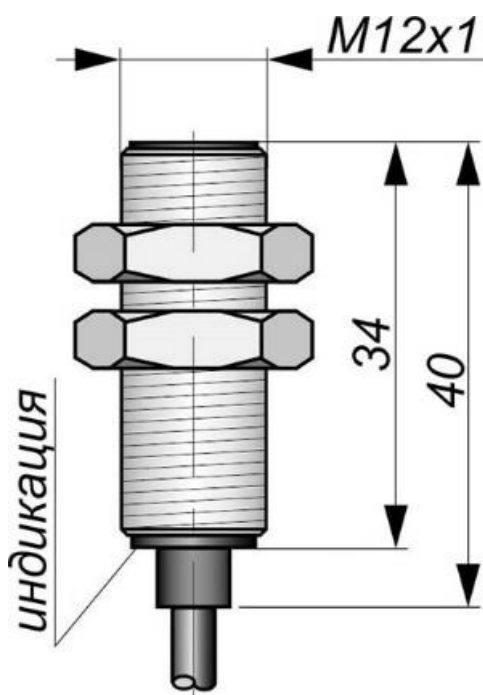
Габаритный чертеж
