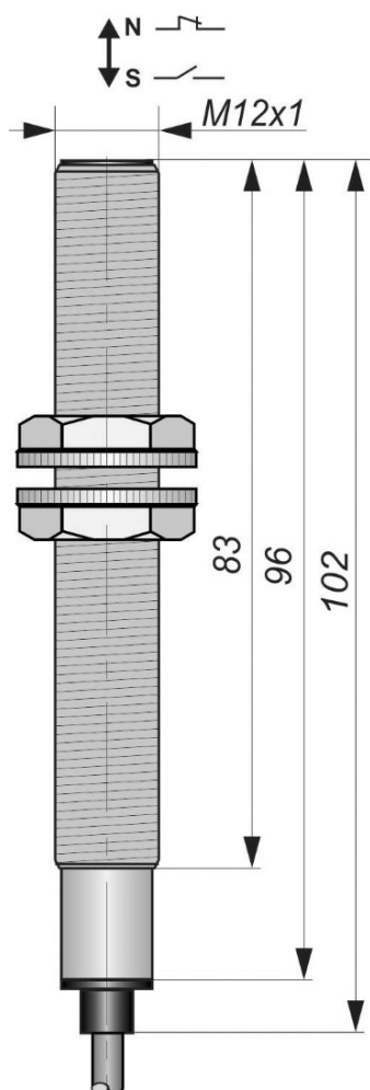
Габаритный чертеж
