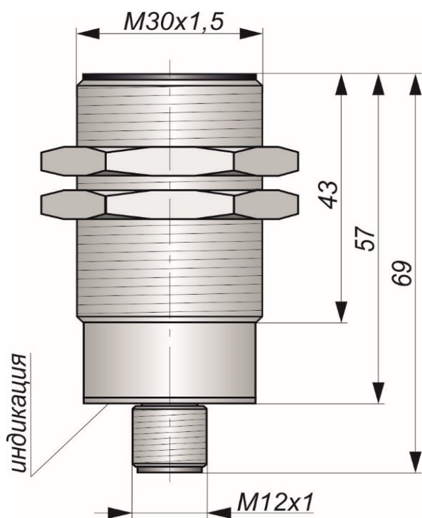
Габаритный чертеж
