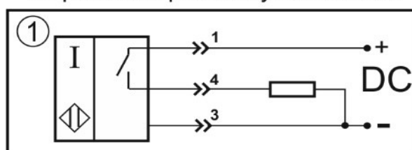
Нормально-разомкнутый контакт
