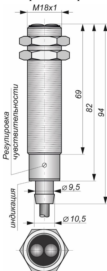
Габаритный чертеж
