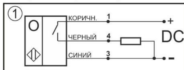
Нормально-разомкнутый контакт
